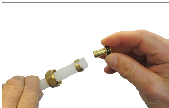
Omløber, klemring og støttebøsning monteres på pexrøret i den nævnte rækkefølge. Koblingen sammenspændes jf. fabrikantens anvisning.
